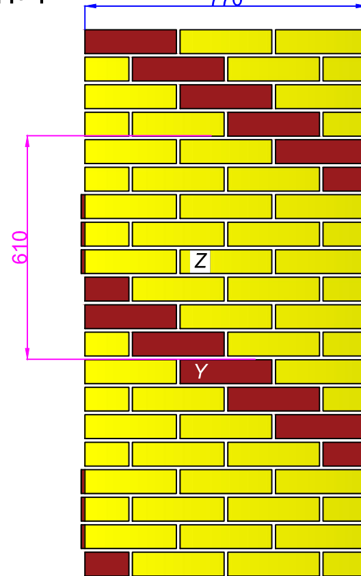
770 Вид-В
